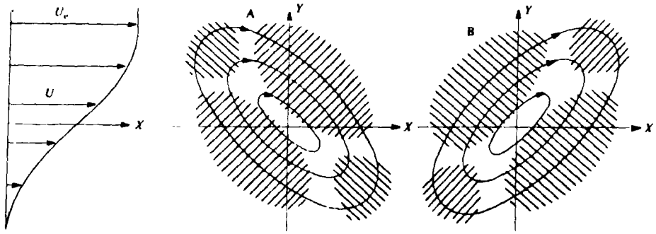
图2 混合边界层中负产生现象
